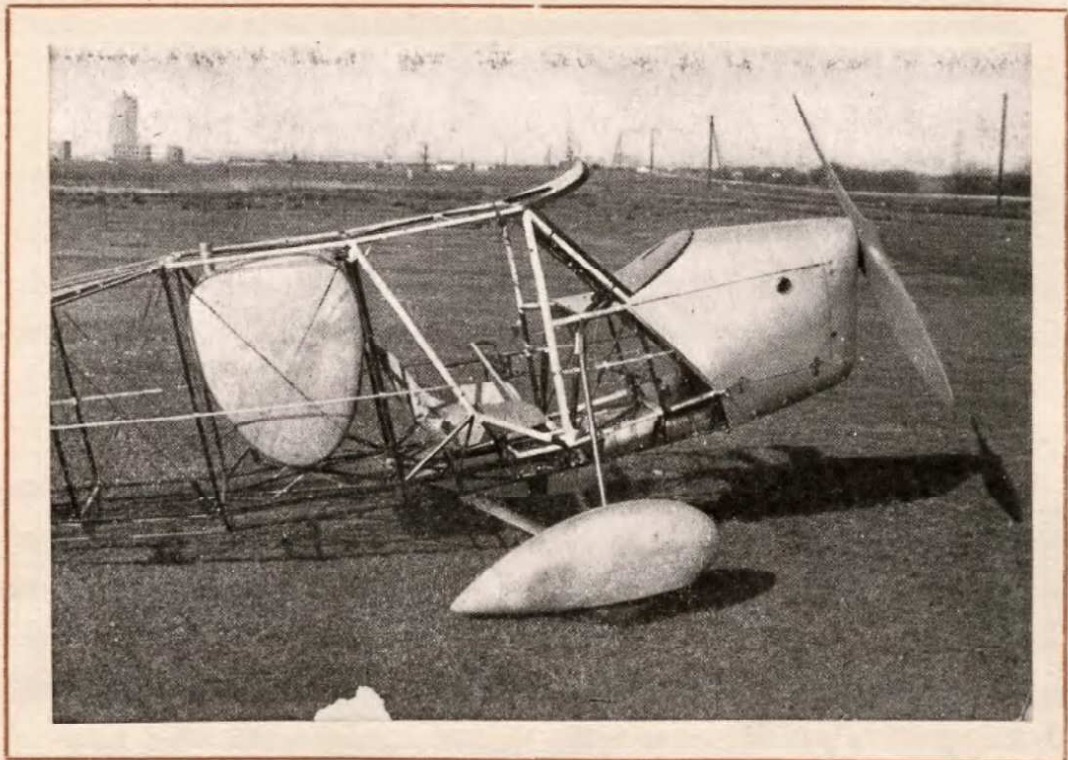
RWD 5-bis w budowie.
